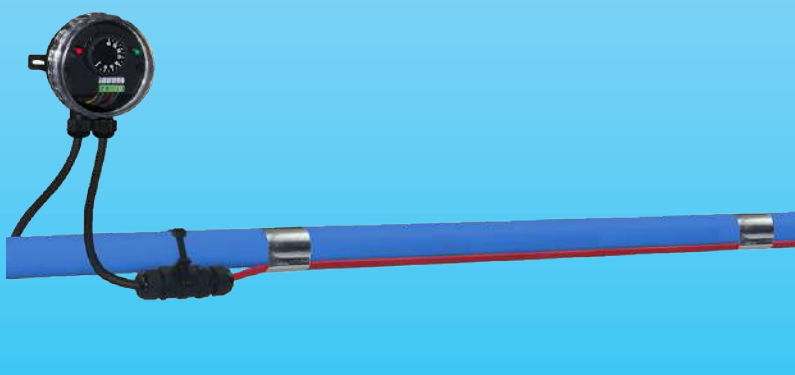
Exemple de montage en commande d'un câble chauffant pour mise hors gel d'un tuyau en PVC, combiné avec un boîtier Y24.
